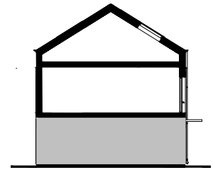
HUSETS SEKTION, ENTRÉPLAN MARKERAT
